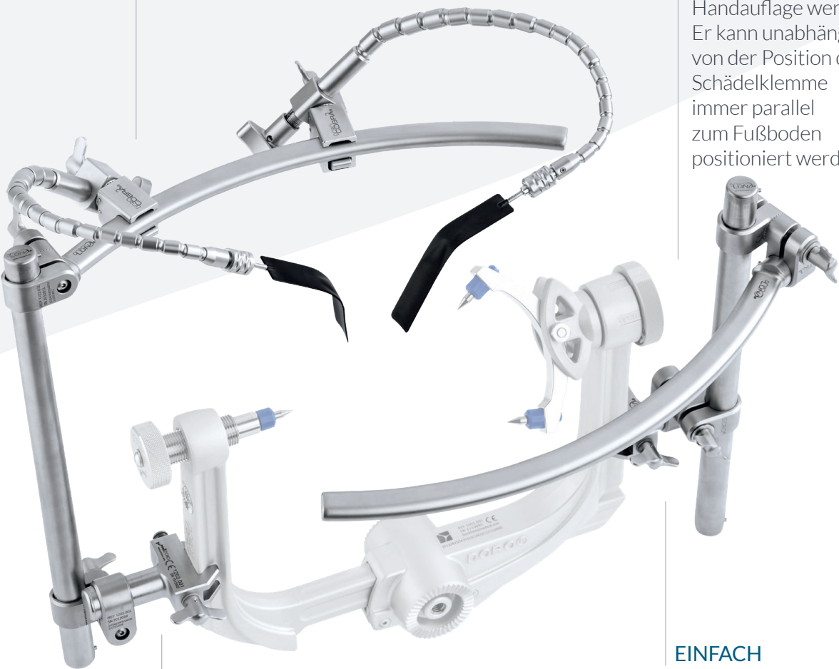
DORO LUNA® Retraktorsystem Standard Artikel-Nr. 1203.100 (auf Abbildung an DORO® QR3-Schädelklemme angebracht)
